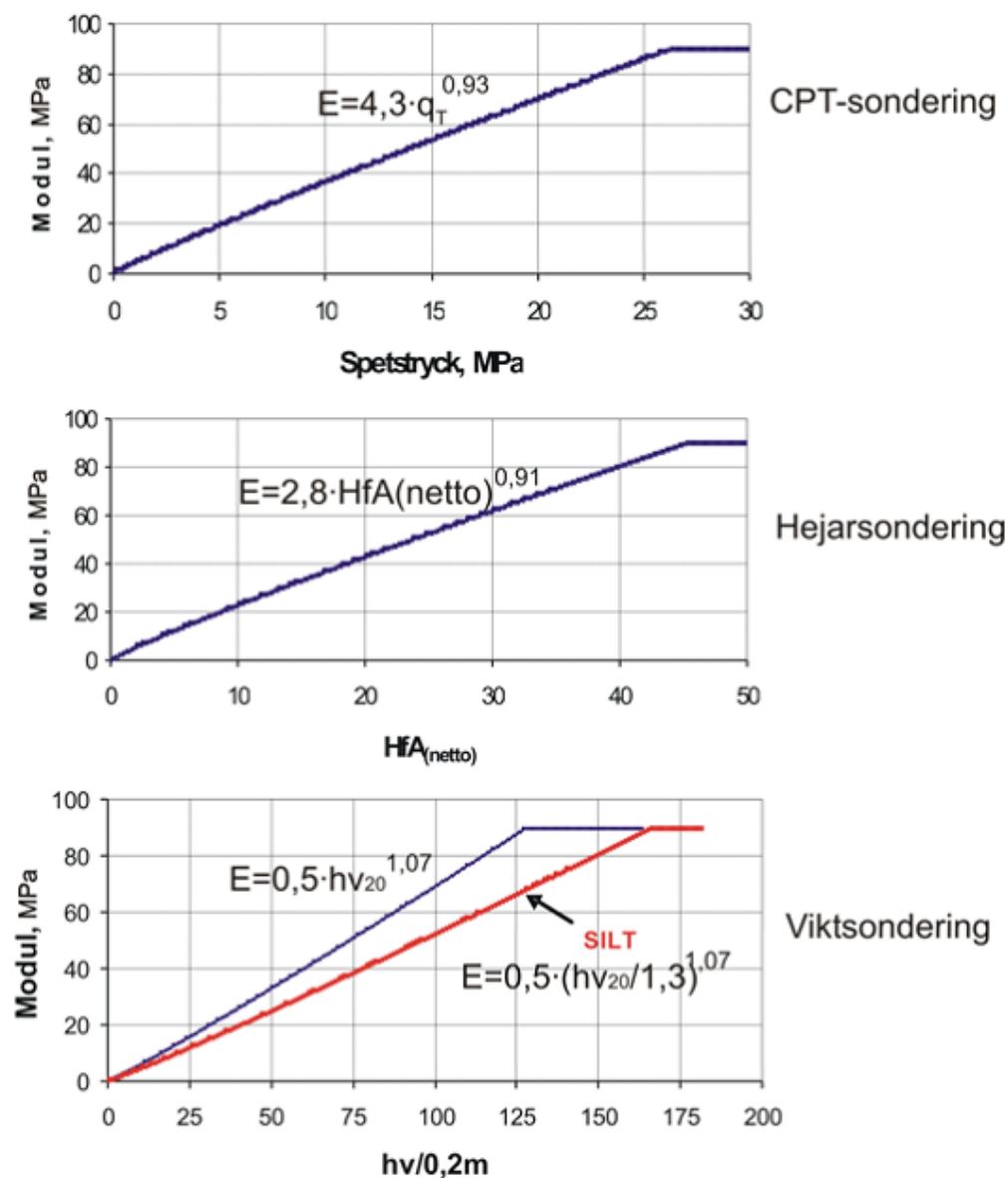
Figur A2-1. Elasticitetsmodul ur sonderingsresultat för sand.
