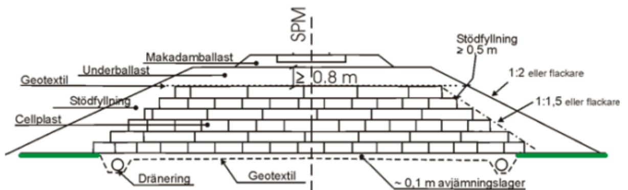
Figur K8.4-2 Bank med cellplast för järnväg.
