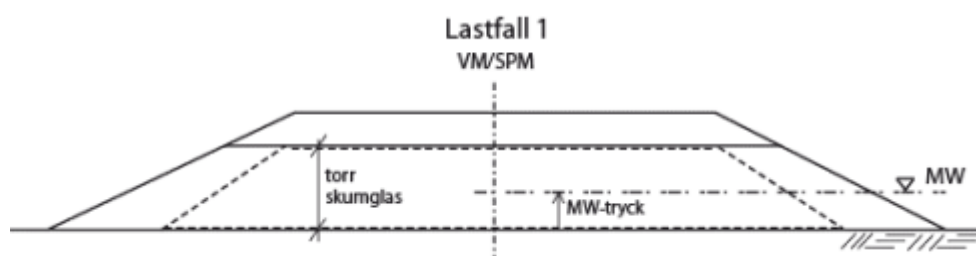
Figur K8.4-6. Lastfall 1 motsvarar nyutlagd skumglas.
