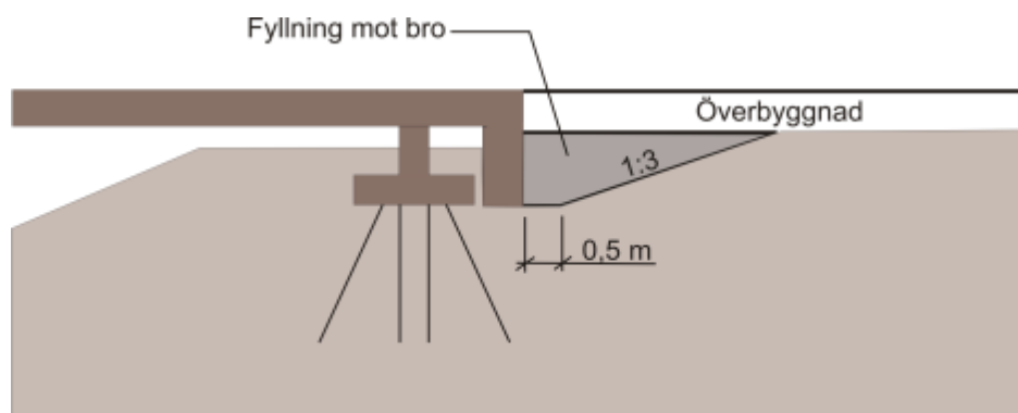
Figur K9.1-2. Fyllning mot ändskärm.
