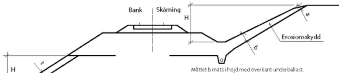
Figur K6.1-2. Utformning av erosionsskydd av jord- och krossmaterial på skärnings- och fyllningslänt.
