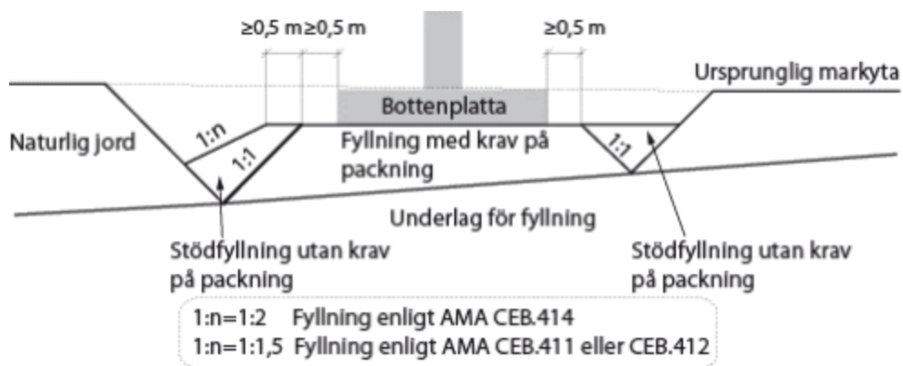
Figur K9.1-1. Packad fyllning för brostöd.
