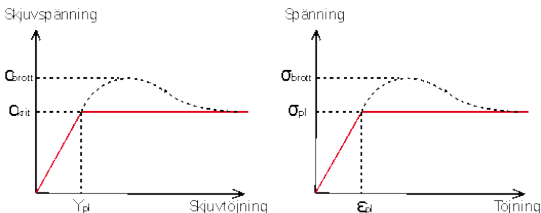
Figur K8.2-1. Spännings-töjningssamband med c_{krit} < 100 kPa. Kritisk skjuvspänning c_{krit} ska antas motsvara 70 % av brottlasten c_{brott} .
