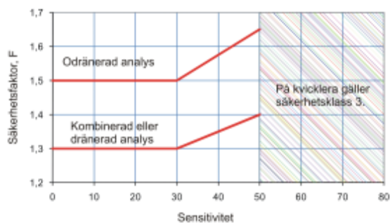
Figur K7.1-2. Lägsta godtagbara totalsäkerhetsfaktor, F_c/F_{c0} , för undergrund av lera i säkerhetsklass 2.
