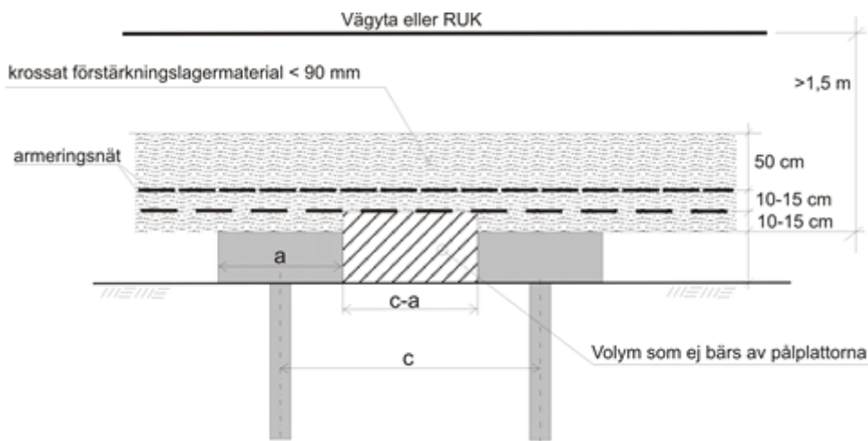
Figur K9.4-2. Principiell utformning av bankpålning med lastfördelande lager med geosyntetisk armering.
