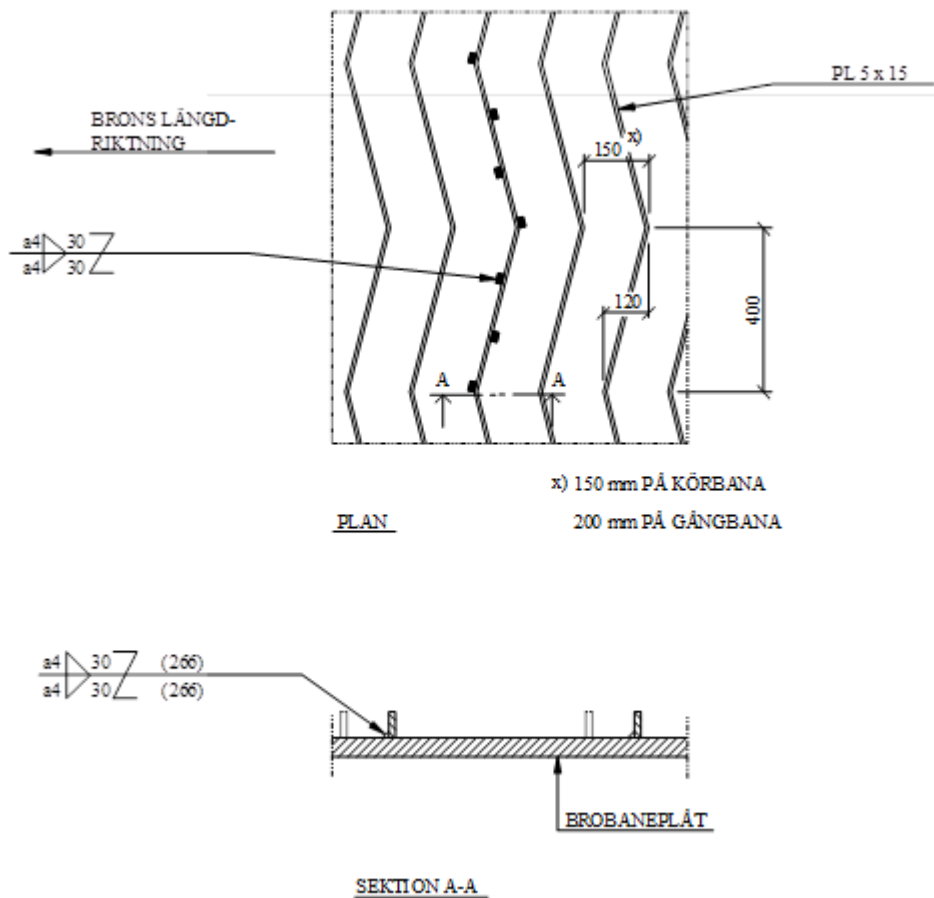
Figur 6.2-5 Sicksackstål på en ortotrop platta till klaffbro
