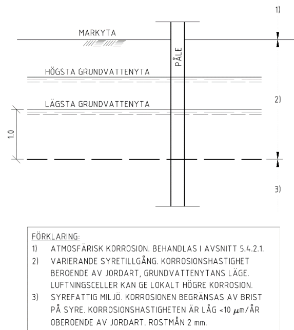
Figur 5.4-1. Beskrivning av pålens olika zoner för val av korrosionsskydd.
